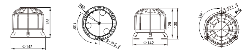
TBD-53X
